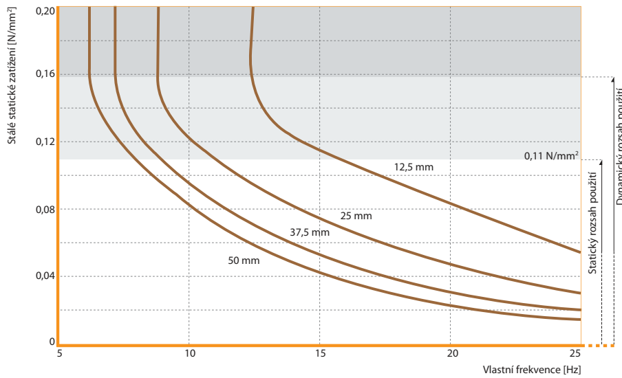
Obr. 3: Vlastní kmitočty volného jednodupňového systému (anglicky „SDOF system“) složený z pevné hmoty a pružné podložky ze Sylomer® SR 110 uložený na tuhém podloží
