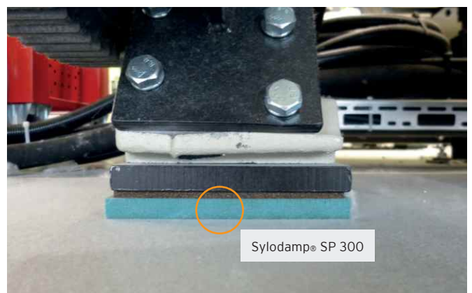
Webmaschinenfuß mit Syloedamp® Lagerung
