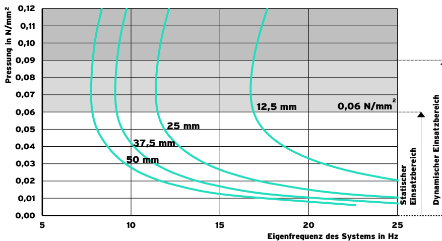
Abb. 3: Eigenfrequenzen eines schwingungsfähigen Systems mit einem Freiheitsgrad, bestehend aus einer starren Masse und einem elastischen Lager aus Relomer® SRG60 auf starrem Untergrund.
