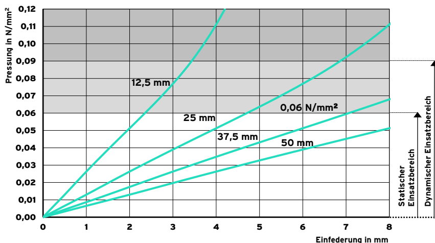
Abb. 1: Quasistatische Federkennlinie mit einer Belastungsgeschwindigkeit von 0,006 N/mm 2 /s.
