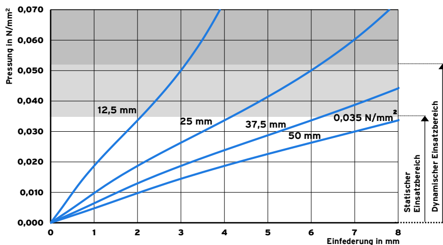
Abb. 1: Quasistatische Federkennlinie mit einer Belastungsgeschwindigkeit von 0,0035 N/mm 2 /s.
