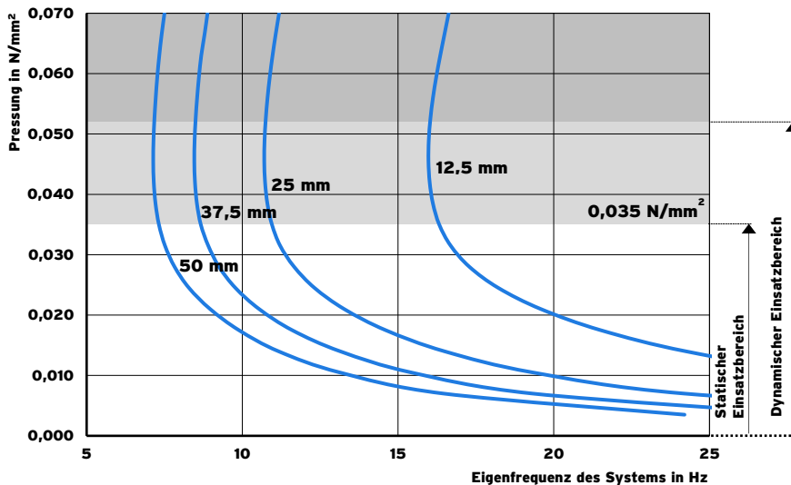
Abb. 3: Eigenfrequenzen eines schwingungsfähigen Systems mit einem Freiheitsgrad, bestehend aus einer starren Masse und einem elastischen Lager aus Relomer® SRG35 auf starrem Untergrund.
