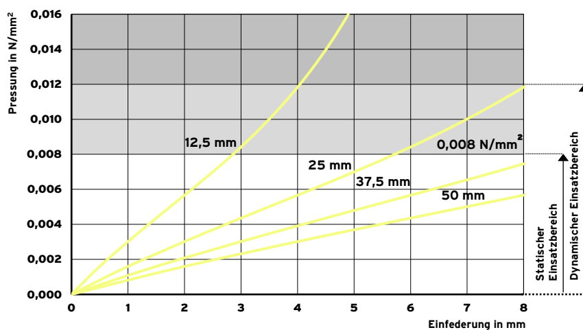
Abb. 1: Quasistatische Federkennlinie mit einer Belastungsgeschwindigkeit von 0,0008 N/mm 2 /s.
