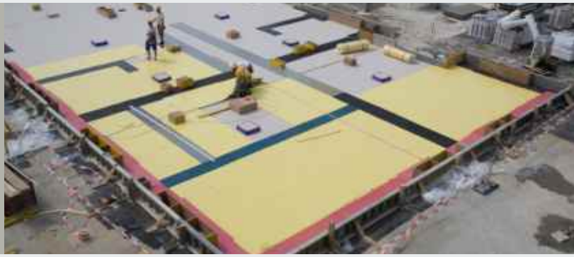
Drachen Center, Basilej, Švýcarsko: celoplošné uložení budovy
