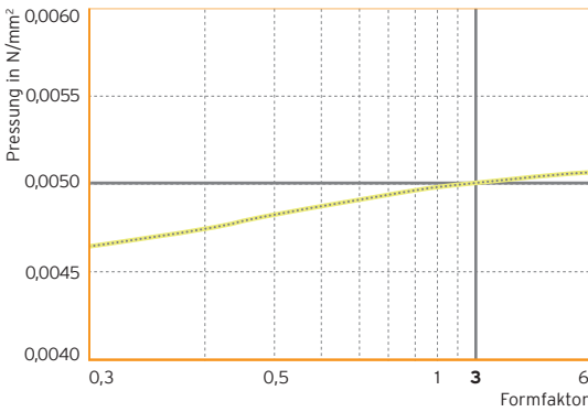
Abb. 5: Statischer Einsatzbereich in Abhängigkeit des Formfaktors
