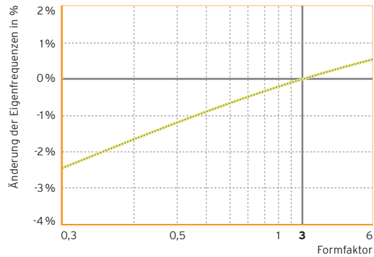
Abb. 8: Eigenfrequenz 5 in Abhängigkeit des Formfaktors
