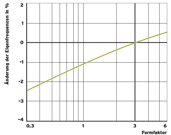
Abb. 8: Eigenfrequenz 5 bei gleichbleibender Dicke in Abhängigkeit des Formfaktors
