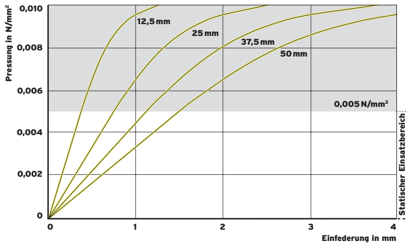
Abb. 1: Quasistatische Federkennlinie für verschiedene Lagerdicken
