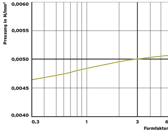
Abb. 5: Statischer Einsatzbereich in Abhängigkeit des Formfaktors
