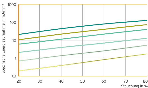
Abb. 9: Energieaufnahme von Syloodamp® bei einer Dicke von 12,5 mm
