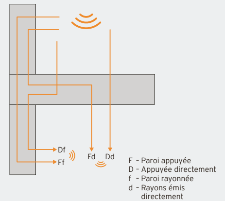
Fig. : Le niveau sonore résulte de la somme des différentes voies de transmission
