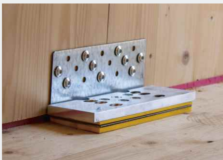
Fig. : Connecteur élastique à angle GEPI Connect 240
