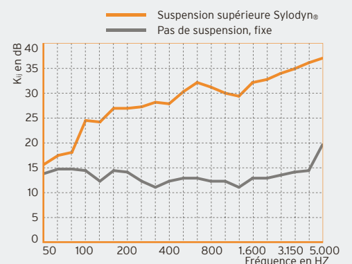
Fig. : Amélioration de la valeur d'isolation de zones de jonction selon la norme EN ISO 10848
