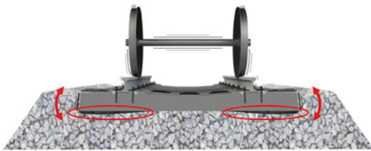
BILD 2: Hohllagenbildung nur unter unbesohnten Betonschwellen. Solche Hohllagen werden durch Schwellenbesohlungen vermieden, was zu einer gleichmäßigeren Lastabtragung führt
