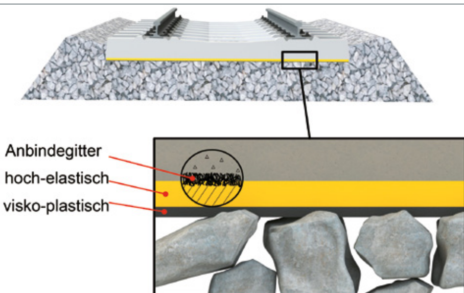
BILD 7: Schwellenbesohlungen im ‚Sandwich-Aufbau‘ mit mehreren funktionalen Schichten
