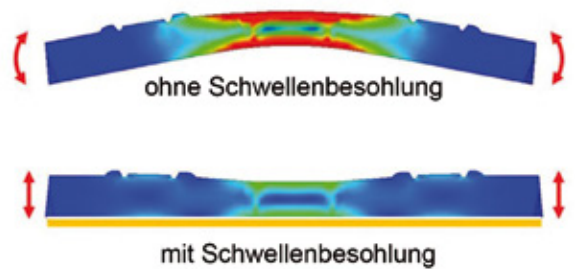
BILD 2: Hohllagenbildung nur unter unbesohnten Betonschwellen. Solche Hohllagen werden durch Schwellenbesohlungen vermieden, was zu einer gleichmäßigeren Lastabtragung führt
