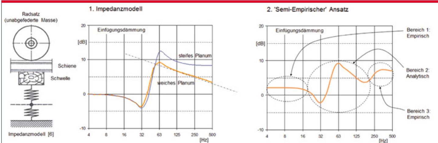
BILD 6: Modellansätze zur Prognose der Einfügungsdämmung von Schwellenbesohlungen
