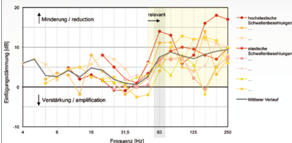
BILD 4: Gemessene Einfügungsdämmungen mit verschiedenen Schwellenbesohlungen
