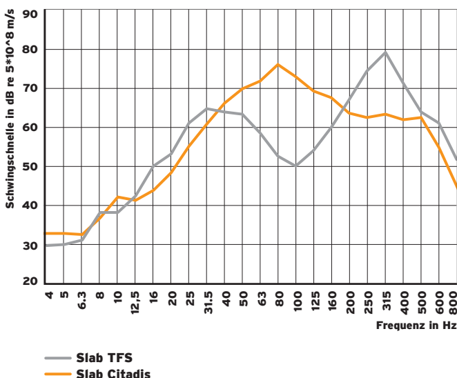
Die eingesetzten Zugtypen TFS und Citadis verursachen bei 63 Hz deutlich unterschiedliche Emissionen...
