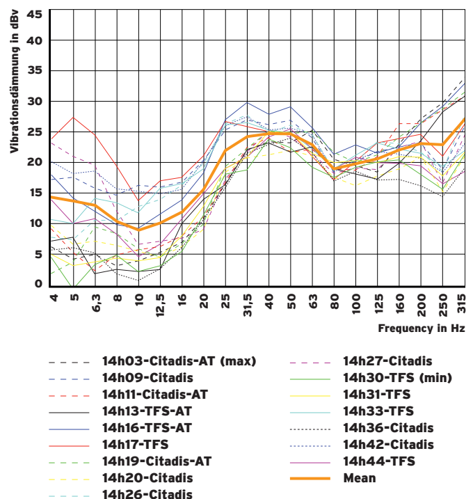
... die mit durchschnittlich 23 dB allesamt zuverlässig vom Getzner-MFS gedämmt werden.
