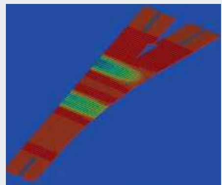
FEM-Modell zur Optimierung der Weichenbesohlung
