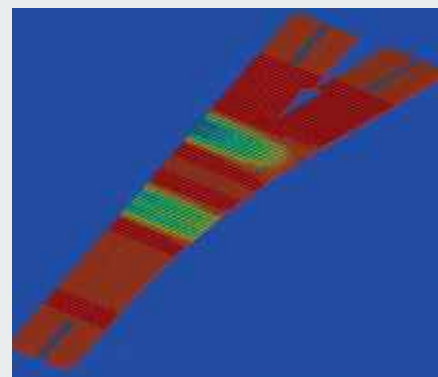
FEM-Modell zur Optimierung der Weichenbesohlung
