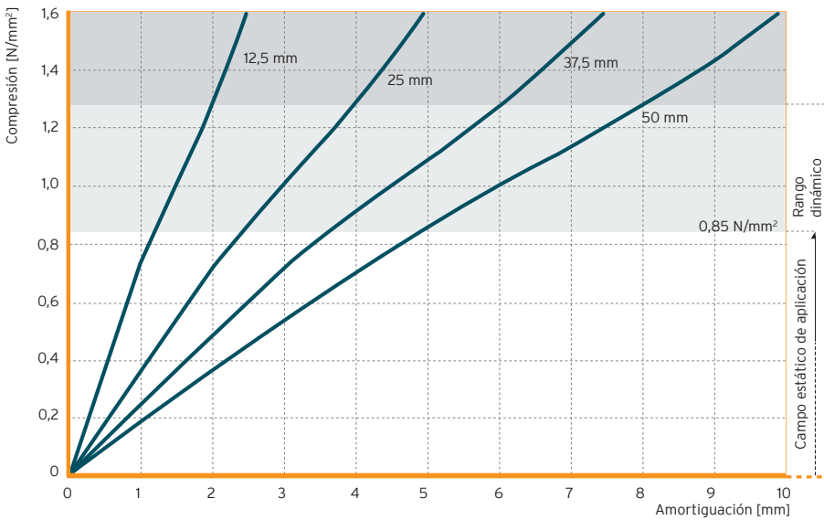
Fig. 1: Curva característica de amortiguación cuasiestática con una tasa de carga de 0,085 N/mm 2 /s
