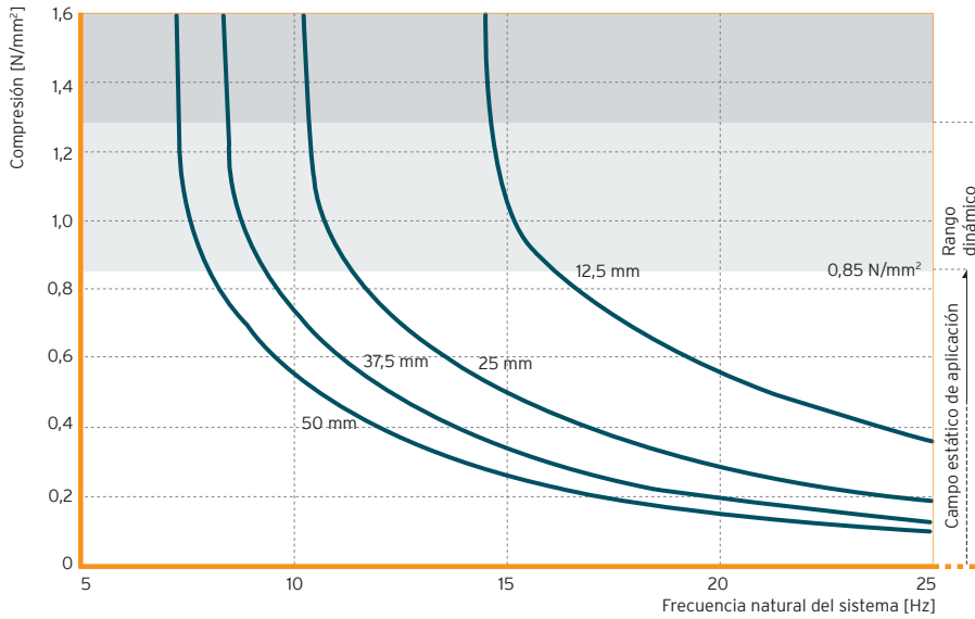
Fig. 3: Frecuencias naturales de un sistema oscilante con un grado de libertad y compuesto por una masa rígida y un soporte elástico de Sylomer® SR 850 sobre base rígida
