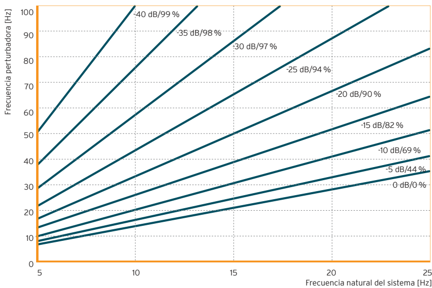
Fig. 4: Reducción de la transmisión de oscilaciones mecánicas mediante la integración de una amortiguación elástica de Sylomer® SR 850 sobre base rígida
