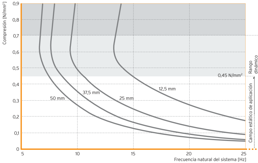
Fig. 3: Frecuencias naturales de un sistema oscilante con un grado de libertad y compuesto por una masa rígida y un soporte elástico de Sylomer® SR 450 sobre base rígida
