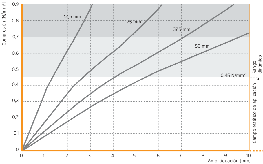
Fig. 1: Curva característica de amortiguación cuasiestática con una tasa de carga de 0,045 N/mm²/s
