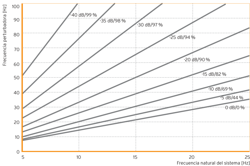
Fig. 4: Reducción de la transmisión de oscilaciones mecánicas mediante la integración de una amortiguación elástica de Sylomer® SR 450 sobre base rígida
