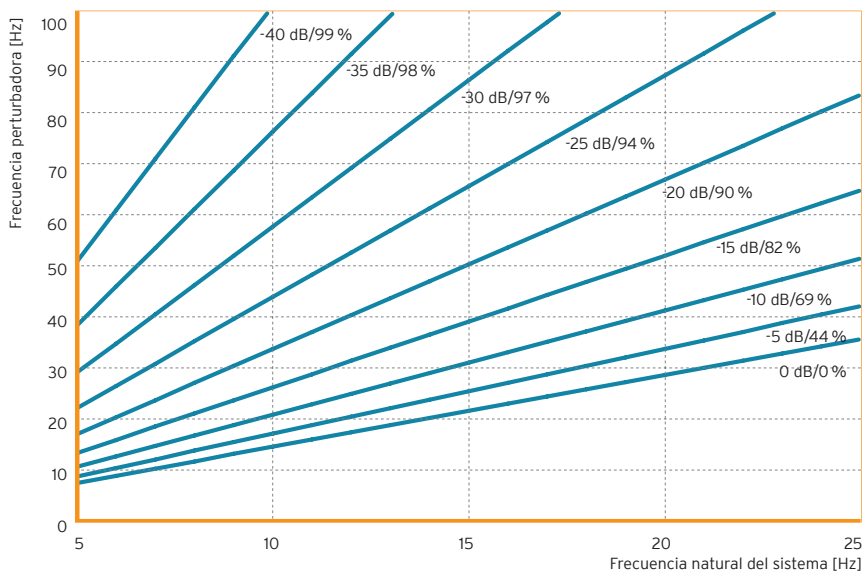
Fig. 4: Reducción de la transmisión de oscilaciones mecánicas mediante la integración de una amortiguación elástica de Sylomer® SR 28 sobre base rígida
