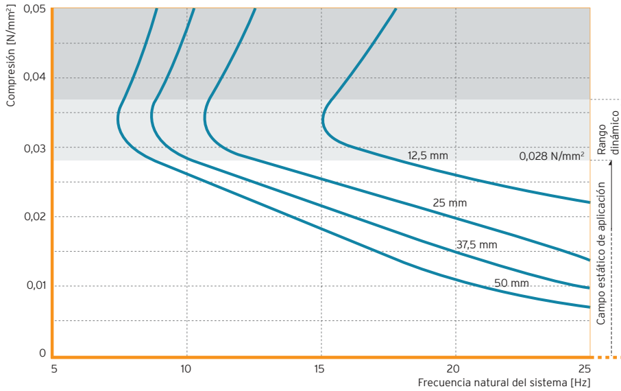
Fig. 3: Frecuencias naturales de un sistema oscilante con un grado de libertad y compuesto por una masa rígida y un soporte elástico de Sylomer® SR 28 sobre base rígida
