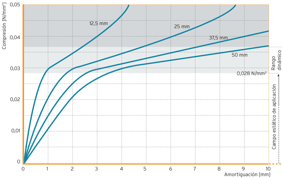
Fig. 1: Curva característica de amortiguación cuasiestática con una tasa de carga de 0,0028 N/mm²/s
