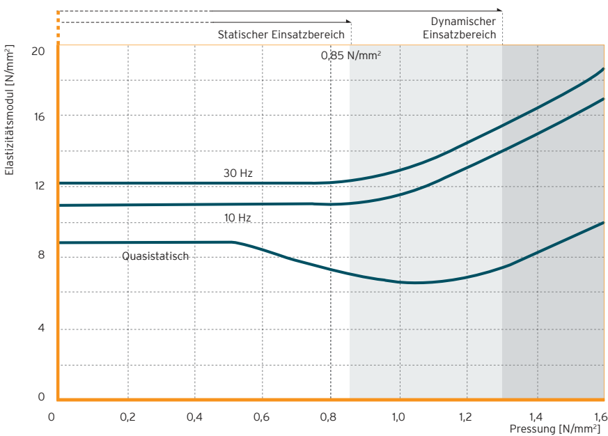
Abb. 2: Belastungsabhängigkeit der statischen und dynamischen Elastizitätsmoduli
