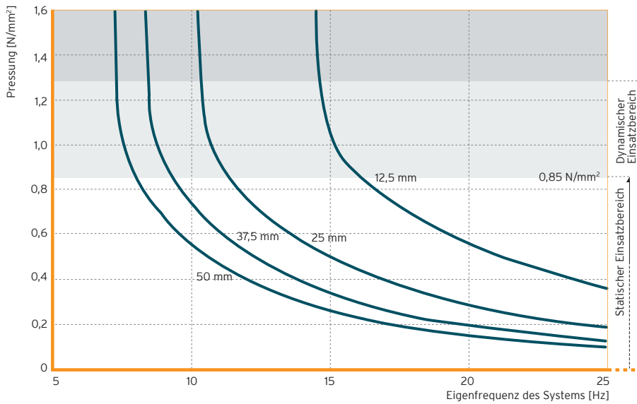
Abb. 3: Eigenfrequenzen eines schwingungsfähigen Systems mit einem Freiheitsgrad, bestehend aus einer starren Masse und einem elastischen Lager aus Sylomer® SR 850 auf starrem Untergrund
