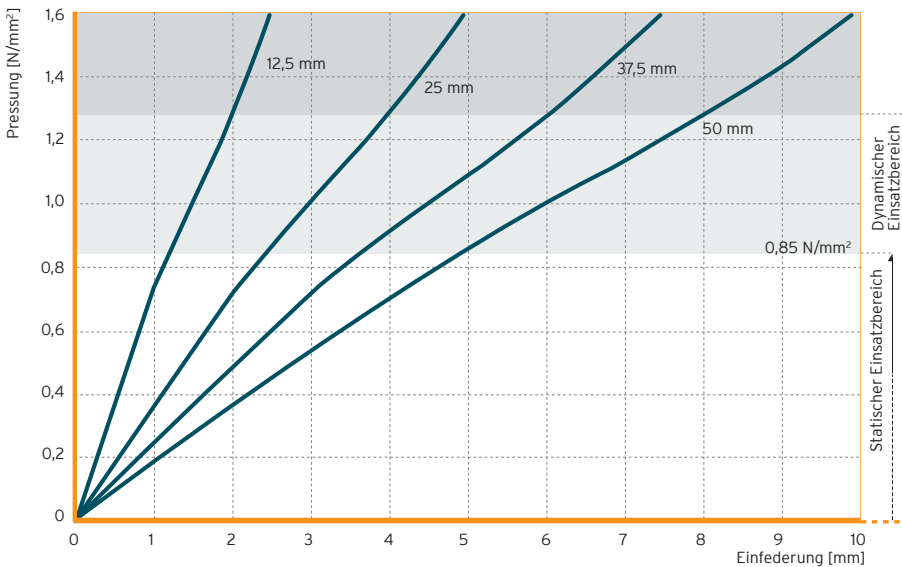
Abb. 1: Quasistatische Federkennlinie mit einer Belastungsgeschwindigkeit von 0,085 N/mm 2 /s
