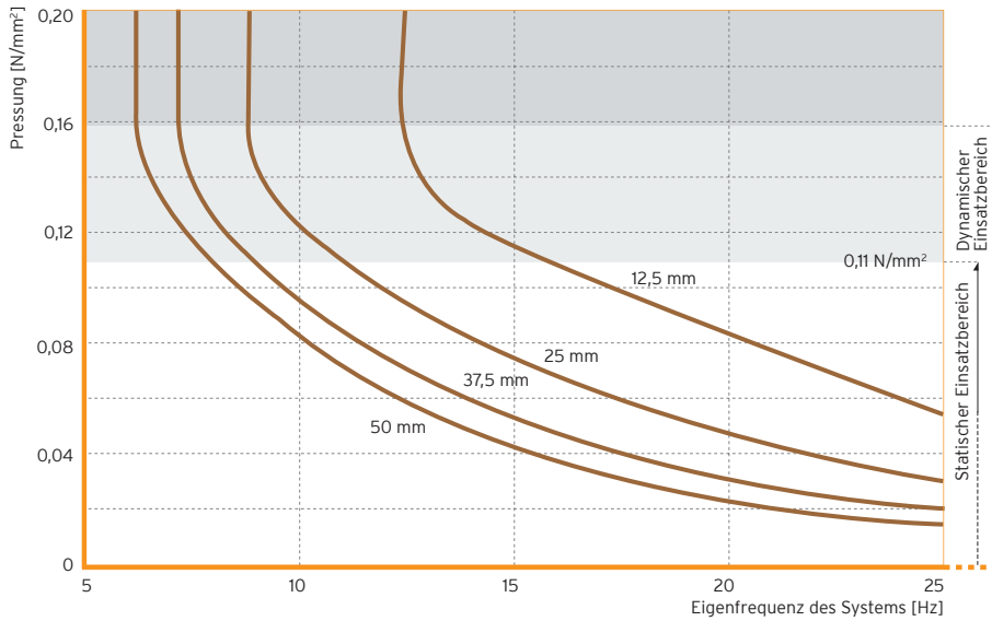
Abb. 3: Eigenfrequenzen eines schwingungsfähigen Systems mit einem Freiheitsgrad, bestehend aus einer starren Masse und einem elastischen Lager aus Sylomer® SR 110 auf starrem Untergrund
