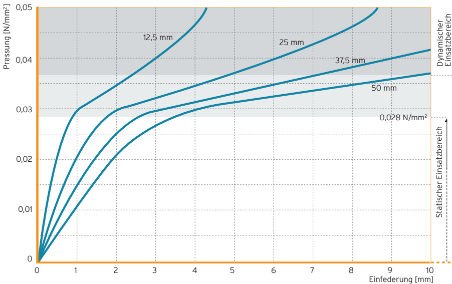
Abb. 1: Quasistatische Federkennlinie mit einer Belastungsgeschwindigkeit von 0,0028 N/mm²/s
