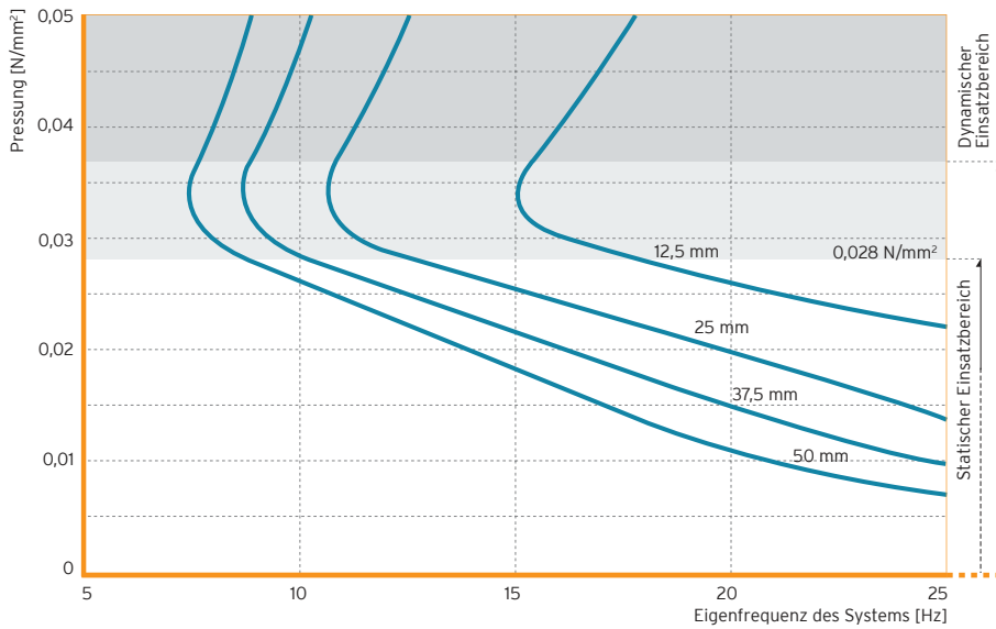
Abb. 3: Eigenfrequenzen eines schwingungsfähigen Systems mit einem Freiheitsgrad, bestehend aus einer starren Masse und einem elastischen Lager aus Sylomer® SR 28 auf starrem Untergrund
