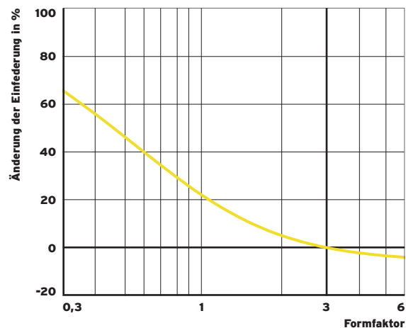
Abb. 6: Einfederung⁴ bei gleichbleibender Dicke in Abhängigkeit des Formfaktors
